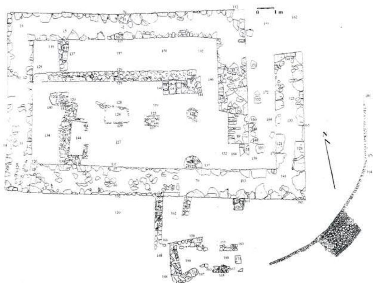
Figura 4. Planimetría del recinto con sus correspondiente cotas y unidades estratigráficas (según Oliver, 2001).
