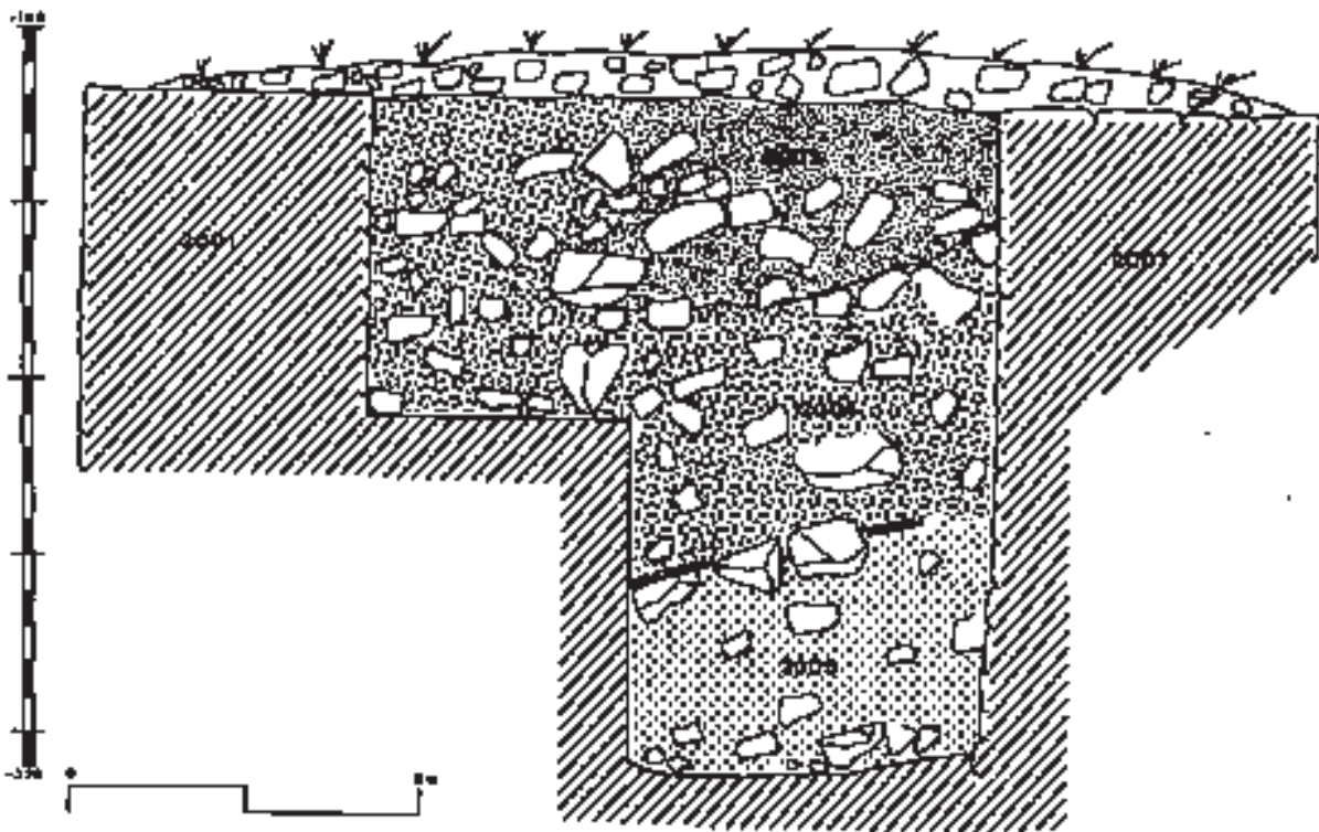
Figura 2. Secció estratigràfica oest-est de l'interior de la torre.
